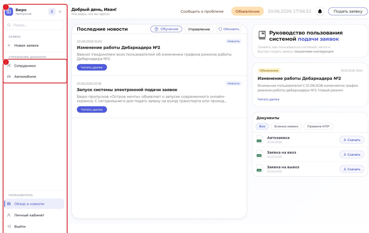
Рисунок 5 — Панель навигации
