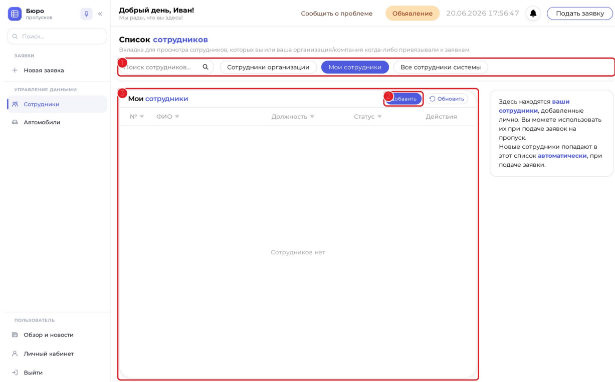
Рисунок 9 — Раздел «Сотрудники»
