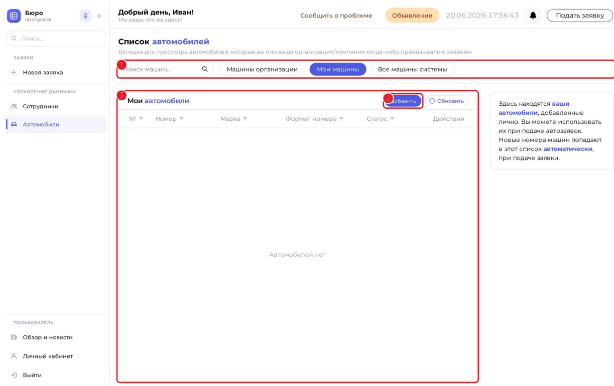
Рисунок 8 — Раздел «Автомобили»
